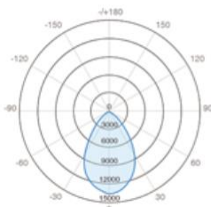
60° Reflector
