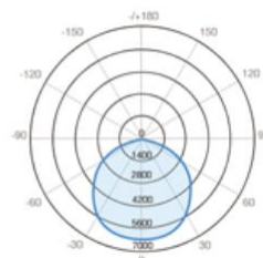
120°, Standard/no Reflector
